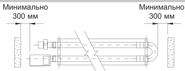
Рис. 26. Инфраизлучатели HELIOS 33S-UD, 50S-UD
