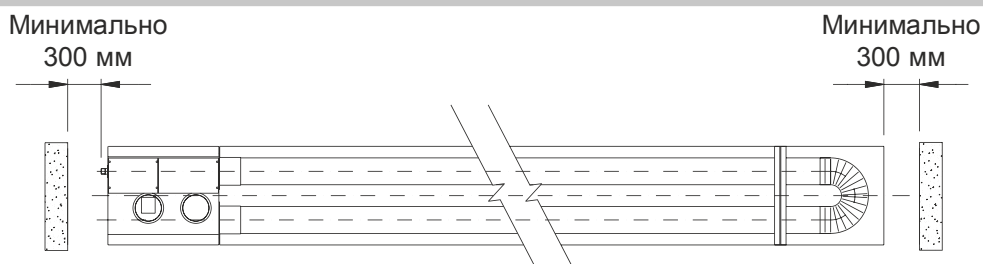
Рис. 26. Инфраизлучатели HELIOS 33S-UD, 50S-UD
