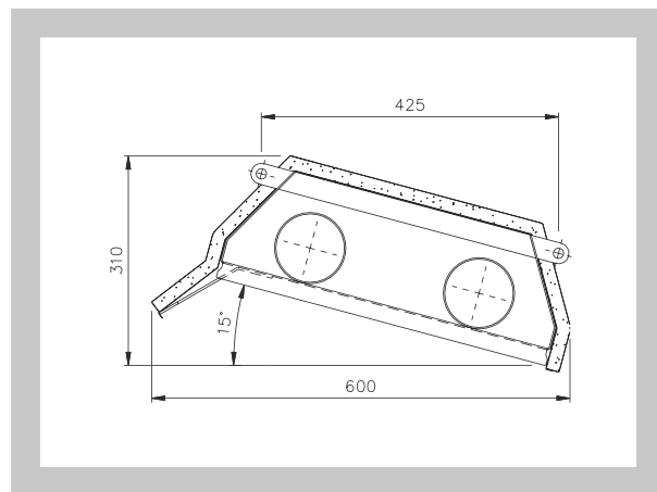
Рис. 4. Сечение отражателя инфракрасных излучателей HELIOS 10 - 50-U/15+, 10 - 50-UD/15+
