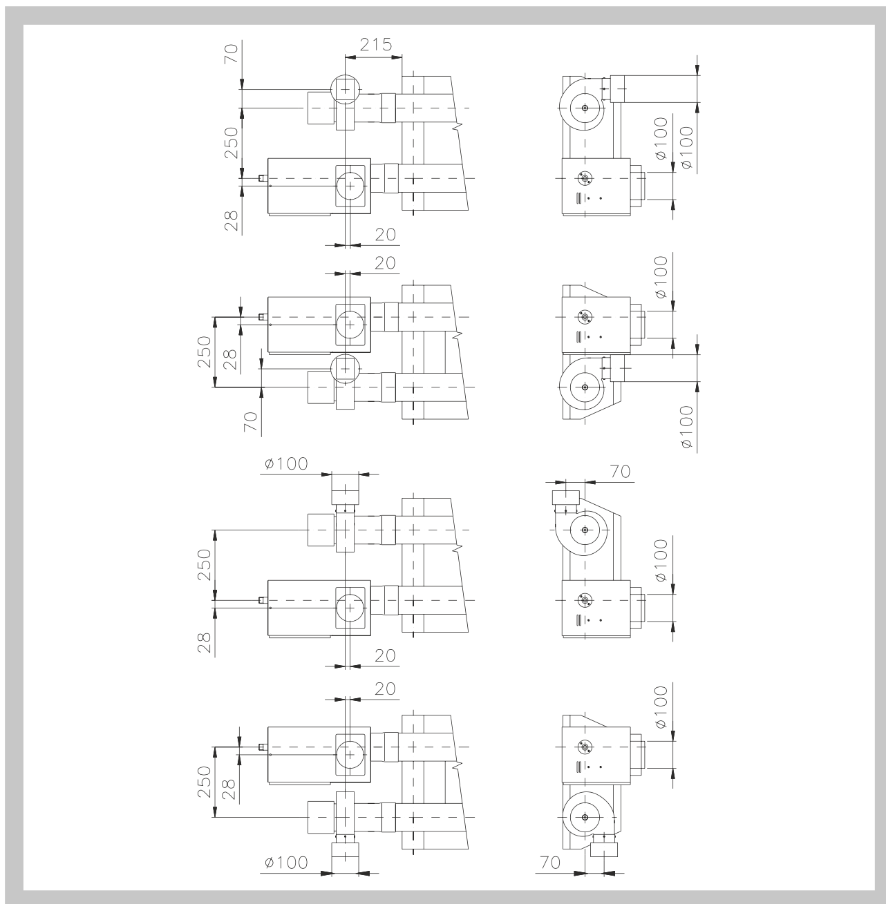
Рис. 21. Положение шкафа горелки и вытяжного шкафа HELIOS 10, 20, 30, 40, 50
