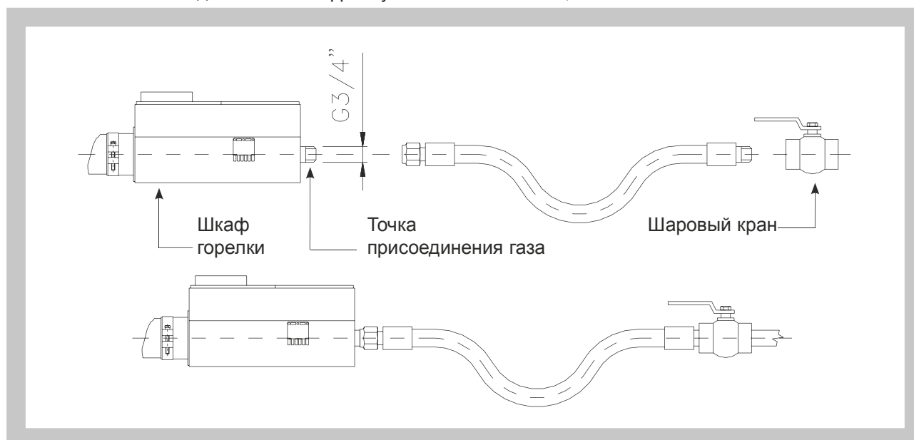
Рис. 30. Точки соединения газинфраизлучатель HELIOS 33S, 50S.
