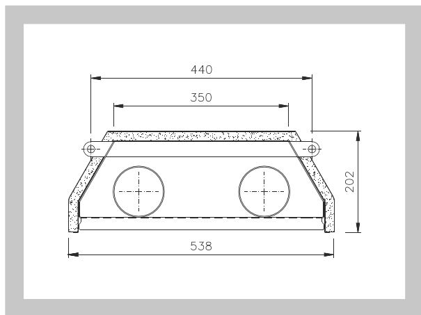
Рис. 3. Сечение отражателя инфракрасных излучателей HELIOS 10 - 50-U+, 10 - 50-UD+
