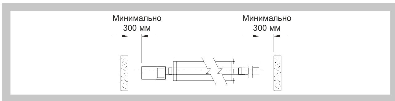
Рис. 27. Инфраизлучатели HELIOS 10 до 40I, 10 до 40ID
