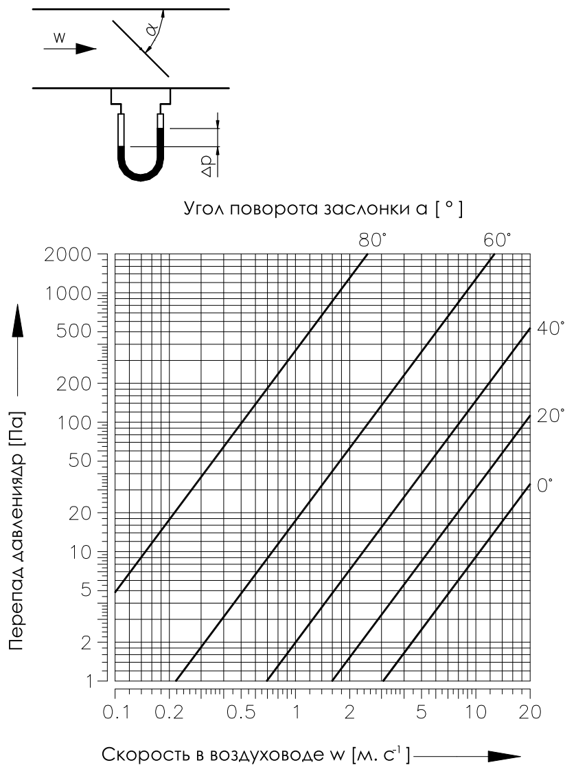
Диагр. 7.1.1. Потери давления в зависимости от положения заслонки
