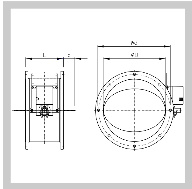
Рис. 4 Заслонка с сервоприводом, фланцевое подключение
