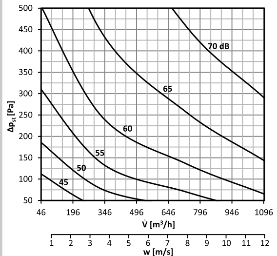
График 8 Уровень акустической мощности L_{WA} [дБ(A)] выделяемой в воздуховод DN180
