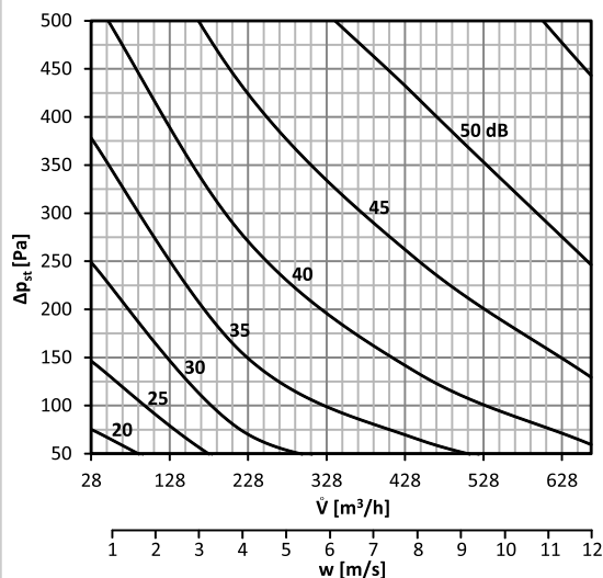
График 19 Уровень акустической мощности L_{wa} [дБ(A)], излучаемой за пределами трубопровода DN180, без изоляции
