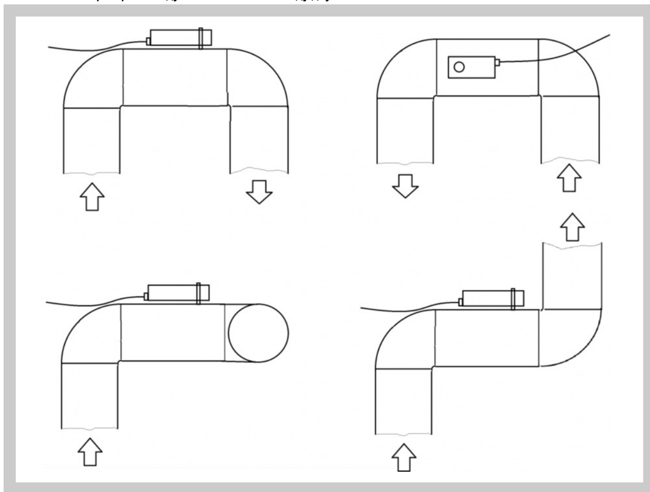
Рис. 9 Некоторые рекомендуемые положения между двумя коленами
