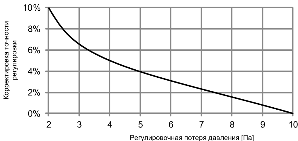
График 2. Корректировка точности регулировки для очень малой регулировочной потери давления
