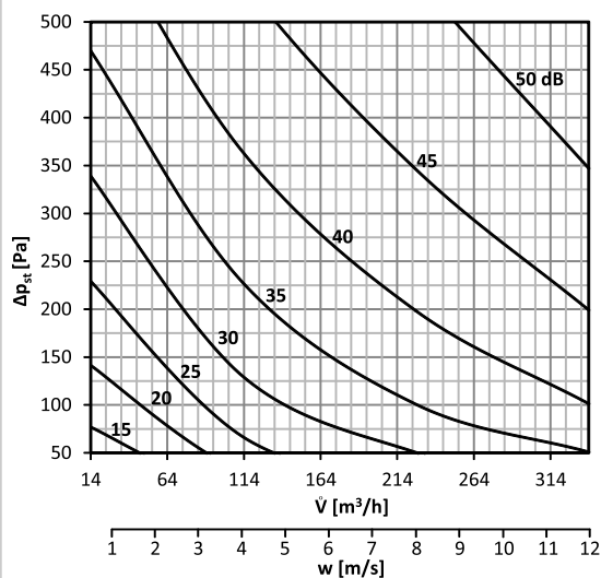
График 17 Уровень акустической мощности L_{wa} [дБ(A)], излучаемой за пределами трубопровода DN150, без изоляции
