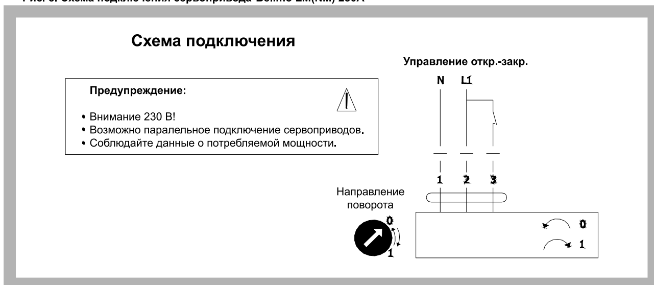
Рис. 8. Схема подключения сервопривода Belimo LM(NM) 230A
