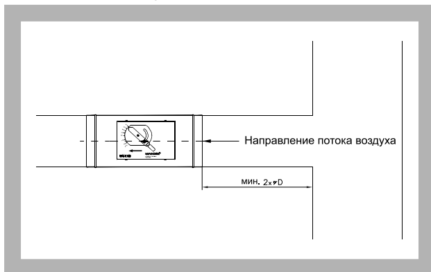
Рис. 6. Рекомендуемое расстояние от разветвления
