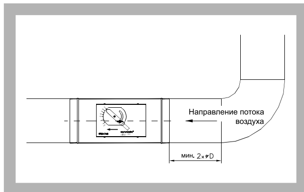
Рис. 7. Рекомендуемое расстояние от изгибов
