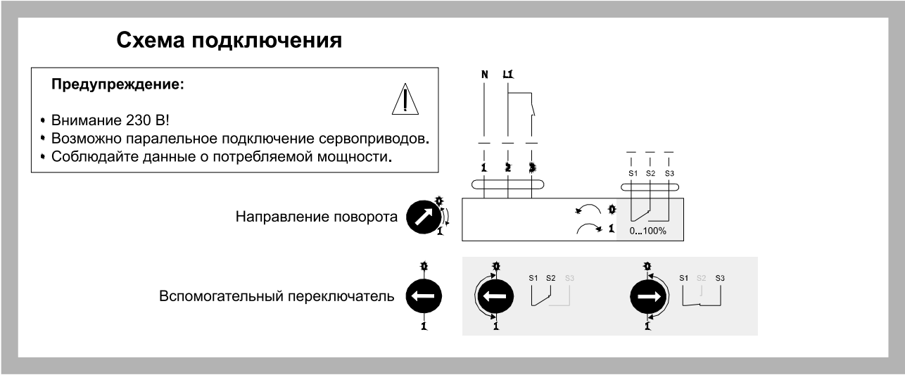
Рис. 11. Схема подключения сервопривода Belimo LM(NM) 230A-S
