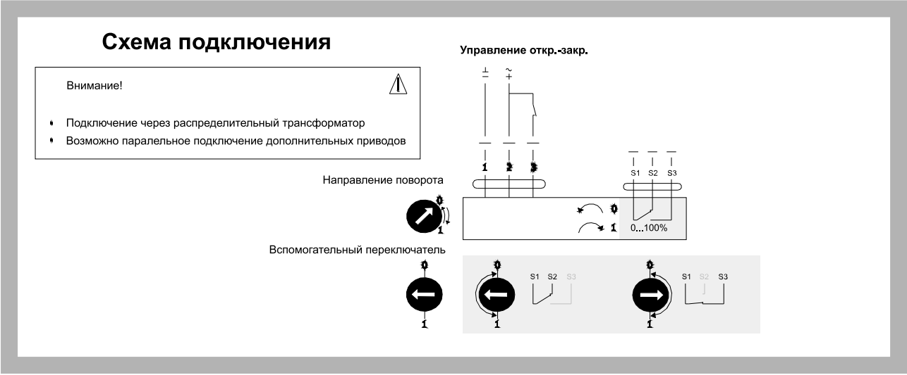
Рис. 12. Схема подключения сервопривода Belimo LM(NM) 24A-S
